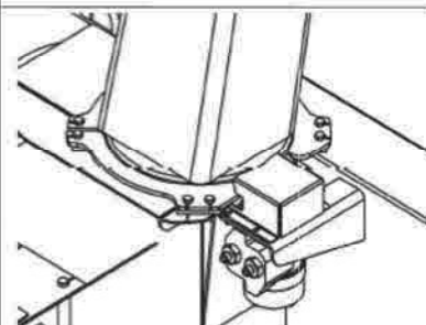
Rotation hydraulique, avec boyaux BER0078A
